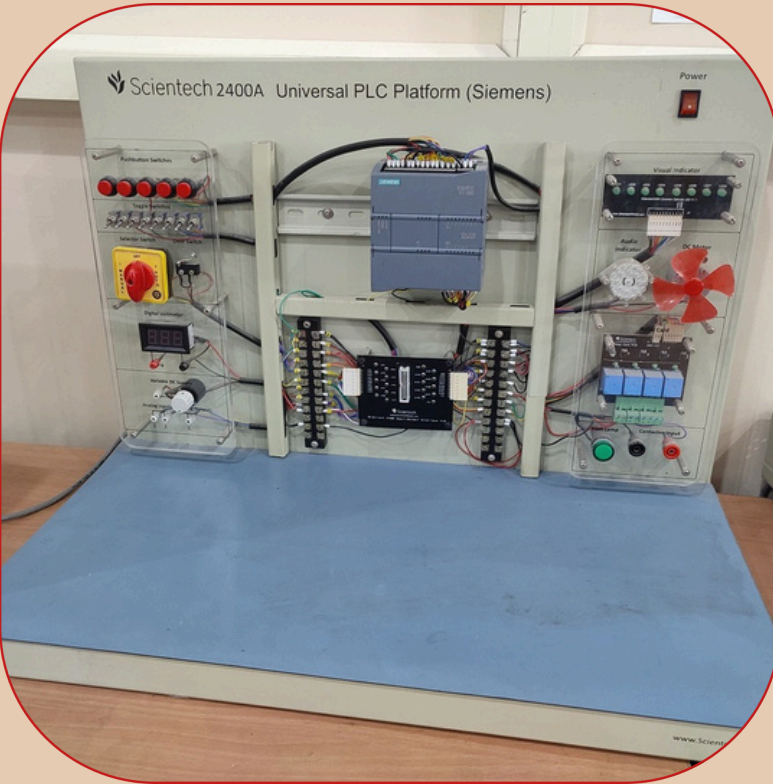
Siemens Sciencetech 2400A Universal PLC Platform (Siemens)
